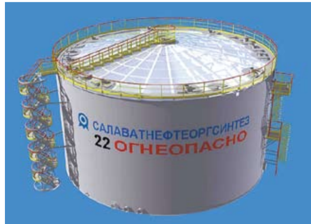
Трехмерная модель реального резервуара поз. Р-22 цеха №13 НПЗ, построенная инженером-конструктором группы архитектурно-строительных сооружений ООО «Салаватгазонефтехимпроект» Андреем Самойловым.
